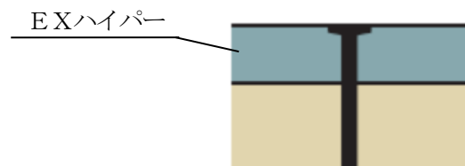
＜釘打ちの概略図＞
